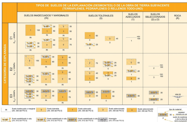
FIGURA 1. FORMACIÓN DE LA EXPLANADA
